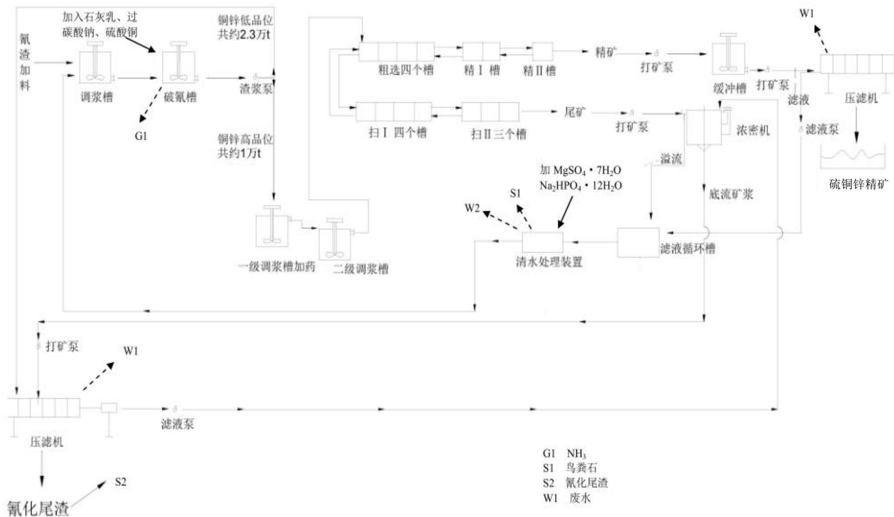
图 3.5-2 氰化尾渣多元素回收工艺流程及产污环节图
